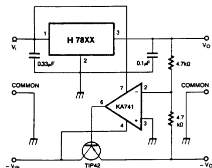
图 10、跟踪稳压器
