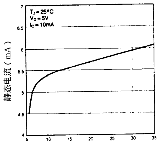
静态电流
