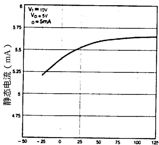
静态电流
